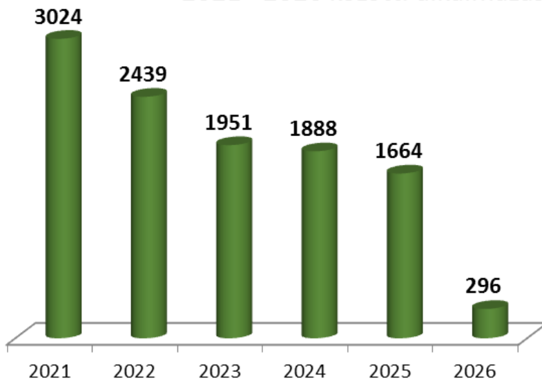
2021 - 2026 közötti alkalmazások
